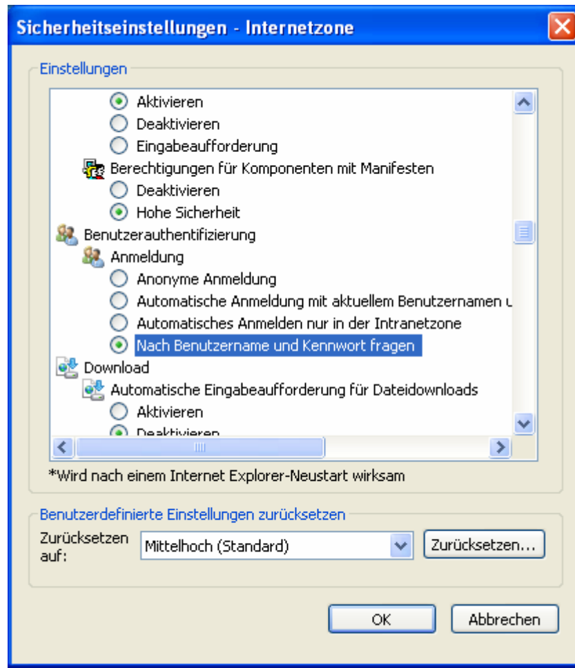
Abb. 5 – Internetoptionen - Internetzone
