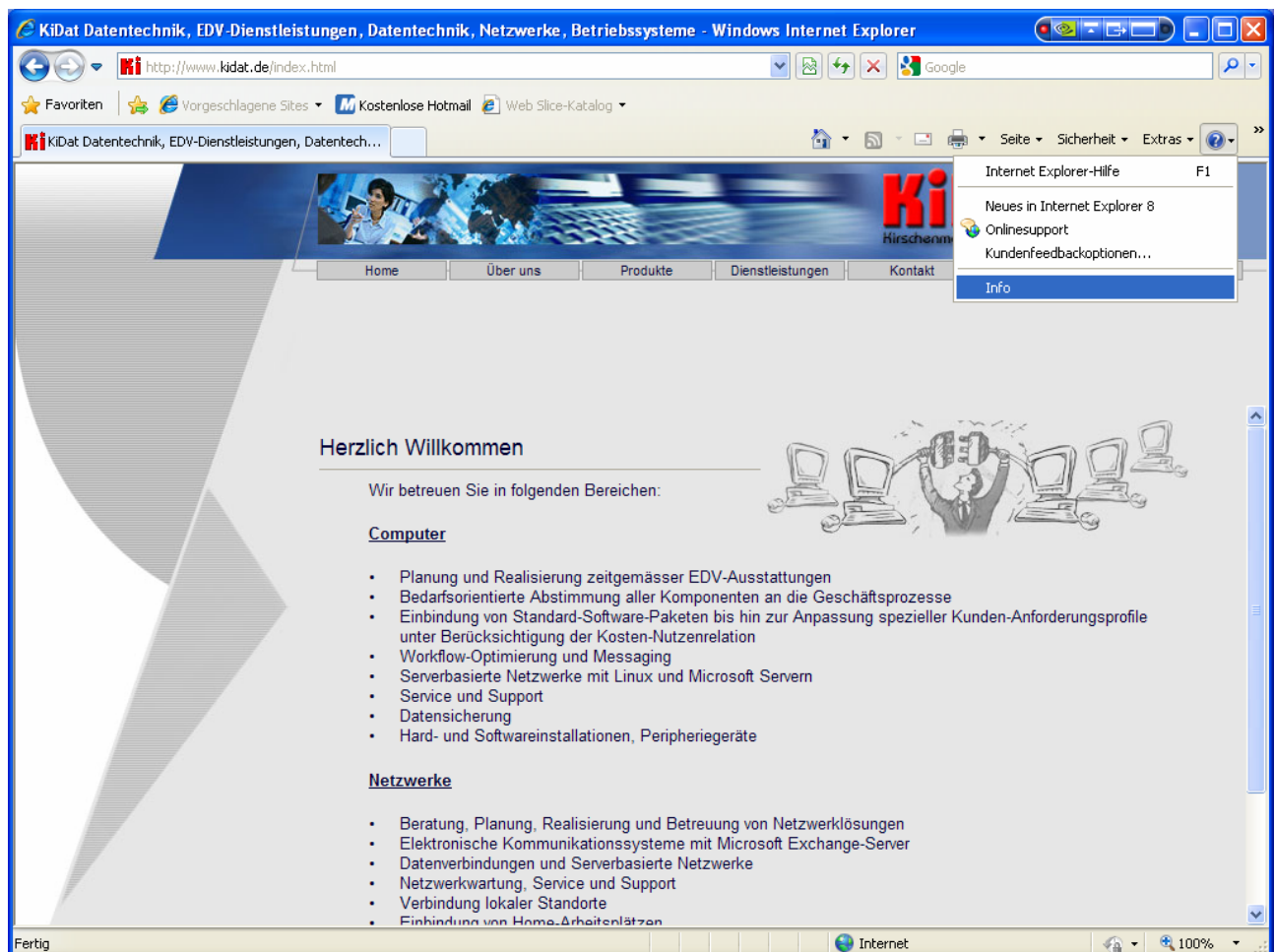
Abb. 1 – Menüpunkt „Fragezeichen“
